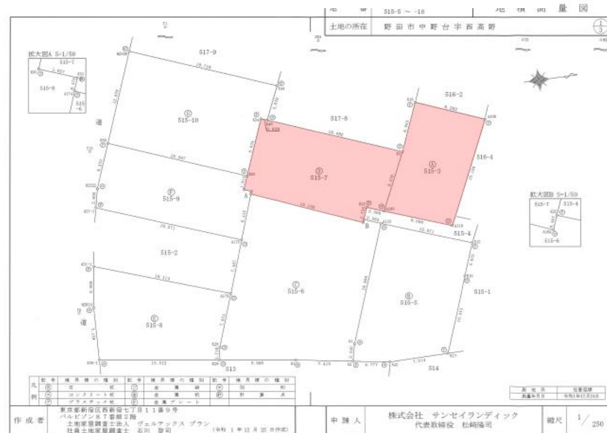
【地積測量図】
