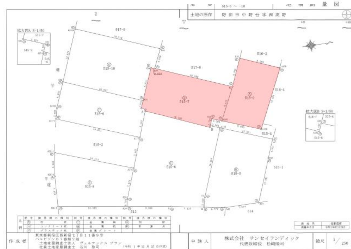
【地積測量図】
