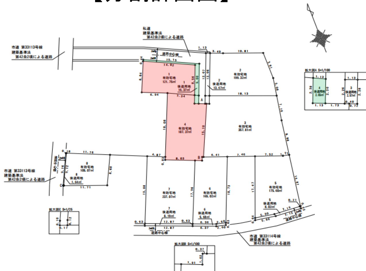
【分割計画図】
